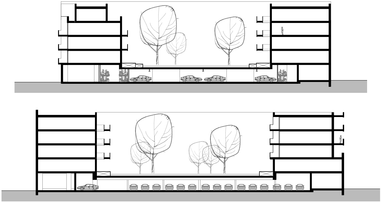
Doorsnedes
