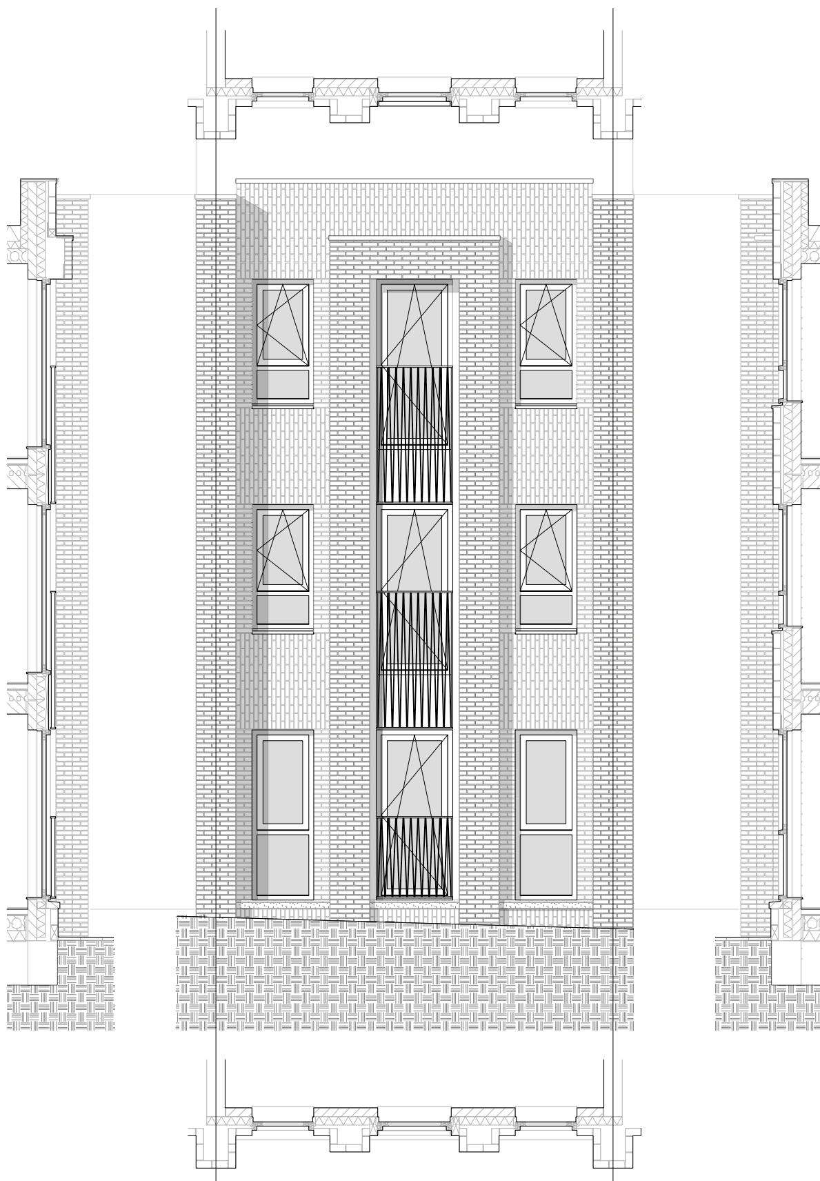
Gevelfragment
