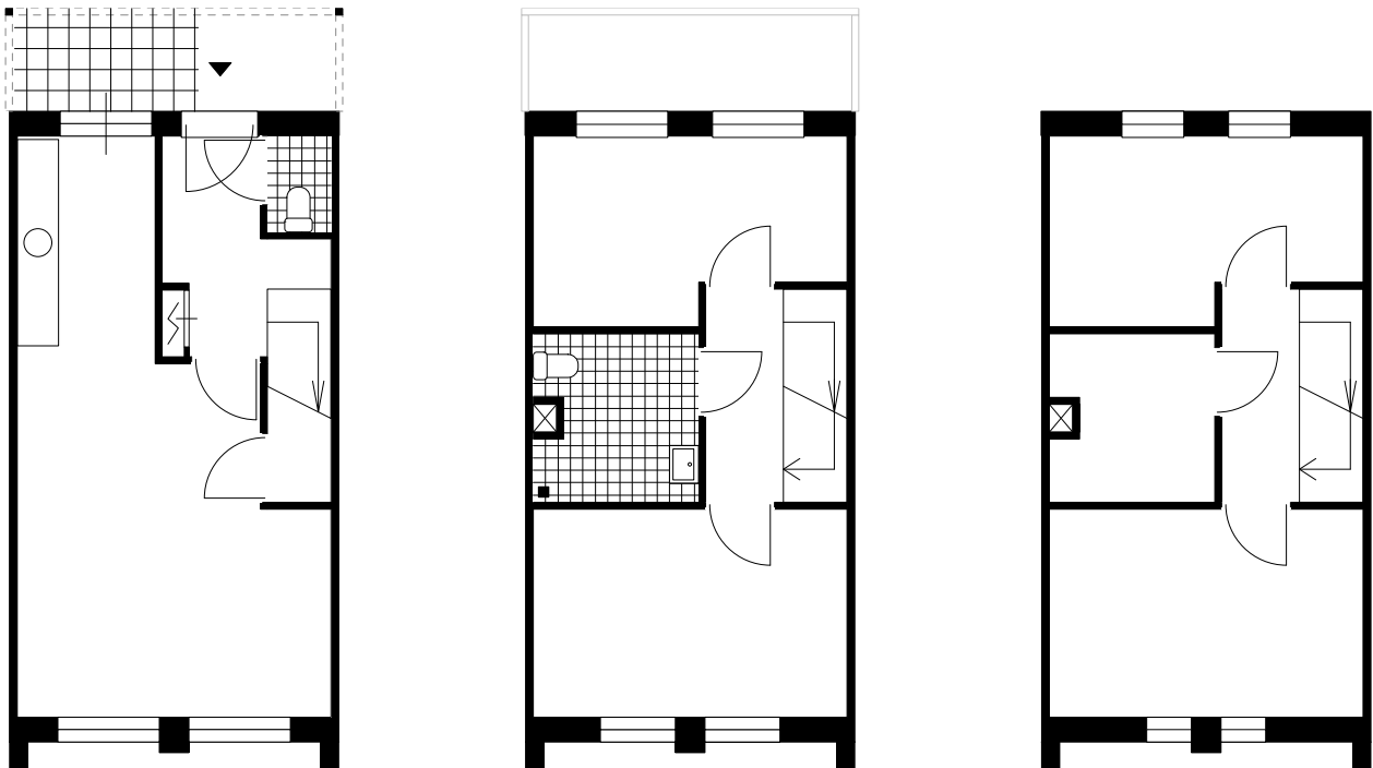
Woningplattegronden eensgezinswoningen: 115 m 2
